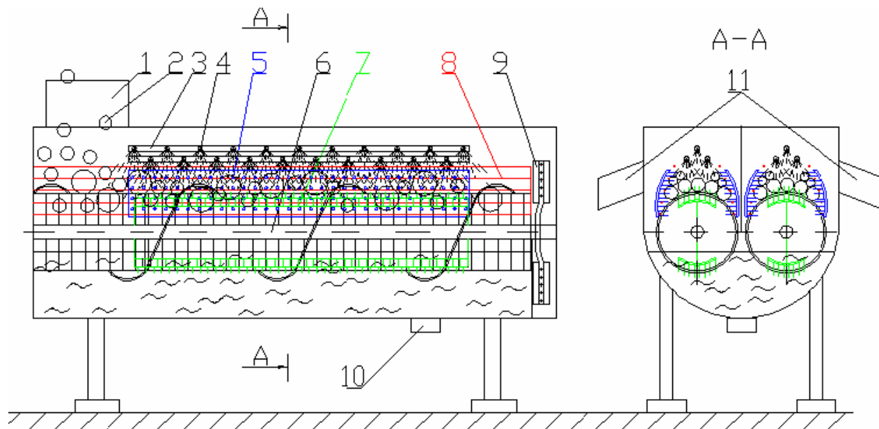
Рис. 2. Схема шнеково-щіткової машини: 1 – завантажувальний лоток; 2 – коренебульбоплоди; 3 – душовий колектор; 4 – форсунка; 5 – щітка (віброюча); 6 – барабан; 7 – щітка; 8 – прутковий кожух; 9 – вивантажувальний механізм; 10 – зливний люк; 11 – вивантажувальні горловини
