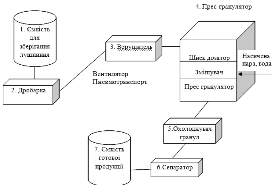
Рис. 1. Схема гранулювання лушпиння
