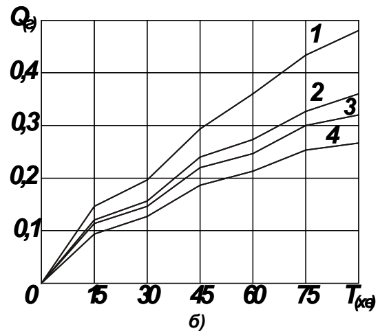
Рис. 2. Залежність зняття металу від тривалості обробки деталей: а) 1 – сталь Ст 3, 2 – сталь 45, 3 – сталь 40х; б) 1 – латунь ЛС601, 2 – сталь 20, 3 – сталь 40, 4 – сталь у8; Умови обробки : A=4^\circ , f=15\text{с}^{-1} , абразив 24А40НСТІ гранули 10÷30
