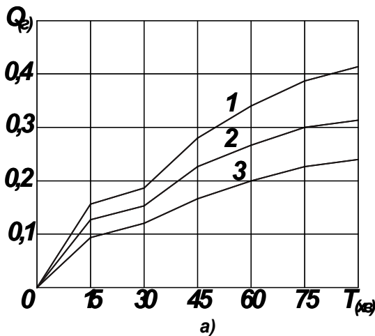
Рис. 2. Залежність зняття металу від тривалості обробки деталей: а) 1 – сталь Ст 3, 2 – сталь 45, 3 – сталь 40х; б) 1 – латунь ЛС601, 2 – сталь 20, 3 – сталь 40, 4 – сталь у8; Умови обробки : A=4^\circ , f=15\text{с}^{-1} , абразив 24А40НСТІ гранули 10÷30
