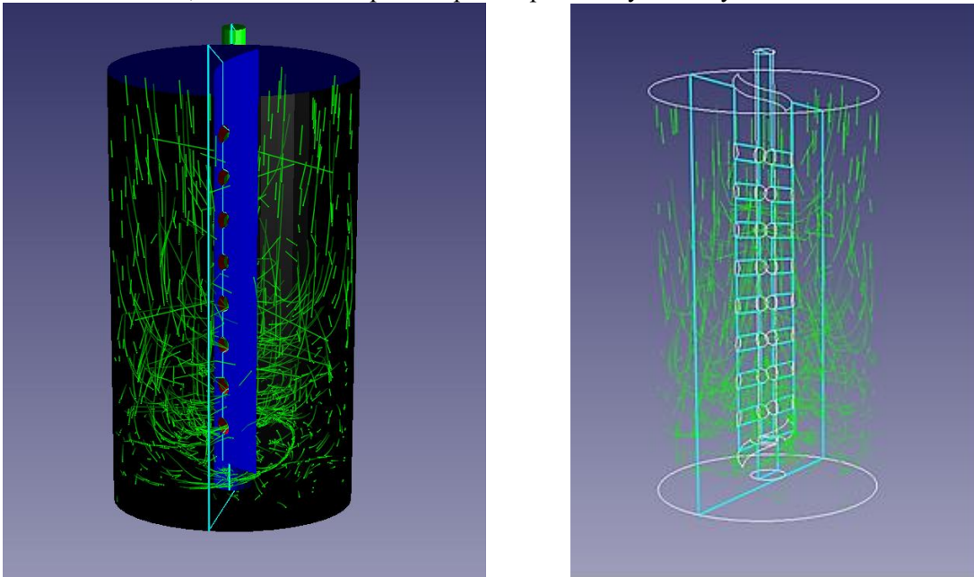
Рис. 1. Моделювання руху потоків палива у змішувачі за допомогою програми FlowVision
