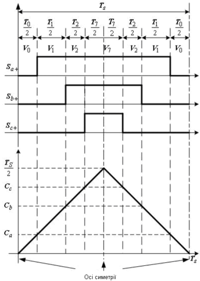
Рис. 4. Осцилограми сигналів керування інвертором і відповідні значення реєстрів порівняння
