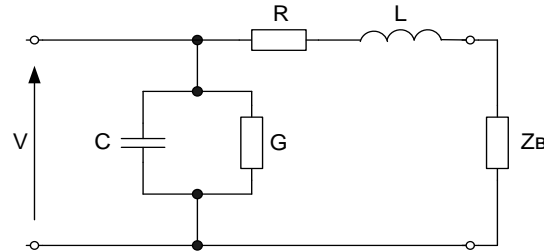
Рис. 5. Електрична схема заміщення смугового несиметричного хвилеводу
