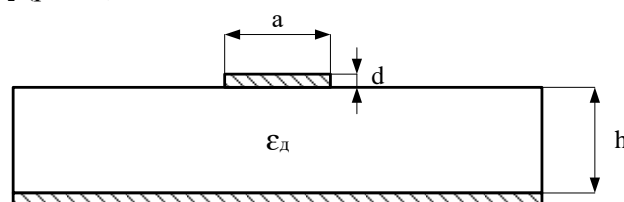
Рис. 3. Поперечний переріз смугового несиметричного хвилеводу
