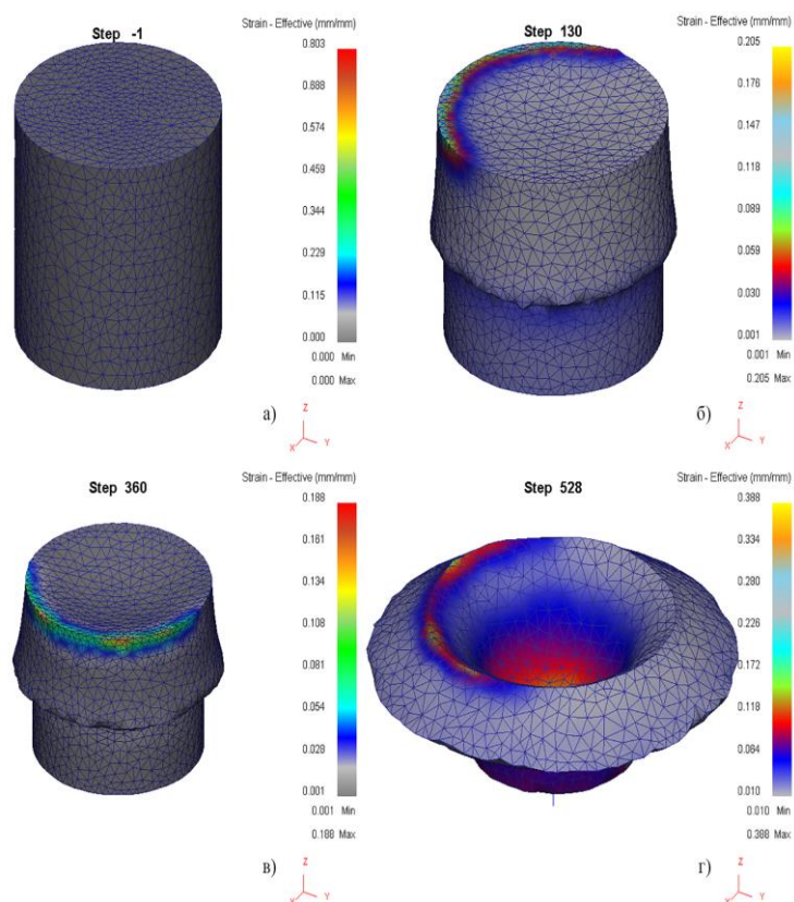
Рис. 1.9. Розподілення інтенсивності напружень по об'єму циліндричної заготовки при ШО: а) початковий етап; б) на 130 кроці ШО; в) на 360 кроці ШО; г) кінцевий крок деформування
