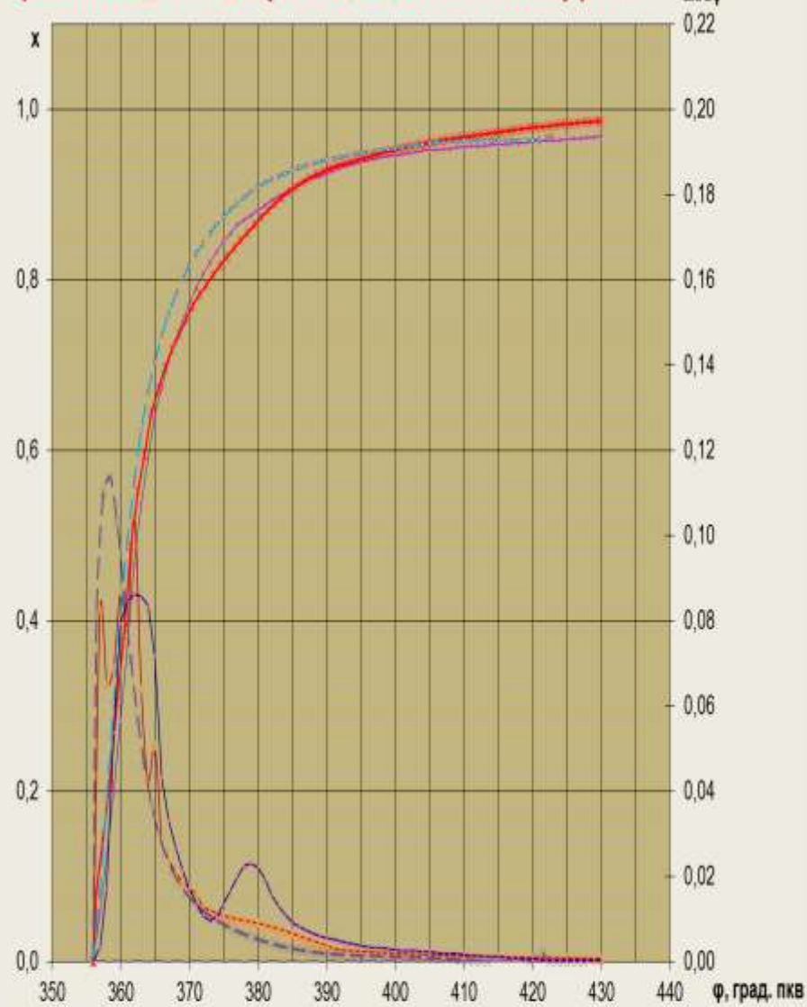
Криві тепловиділення двигуна 4Ч11,0/12,5 на номінальному режимі
