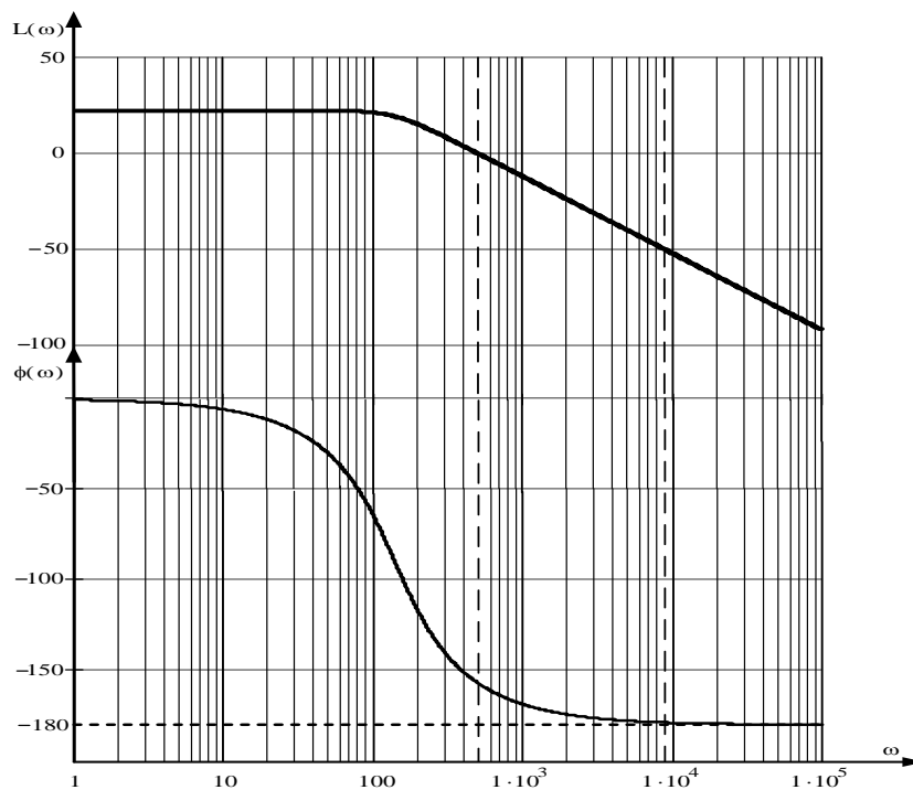
Рисунок 5 – Графіки АЧХ, ЛАЧХ
