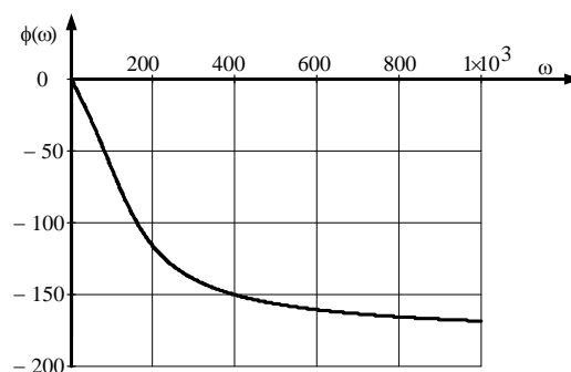
Рисунок 4– Годограф фазочастотної характеристики
