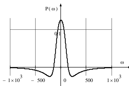
Рисунок 1 – Побудова дійсної частини
