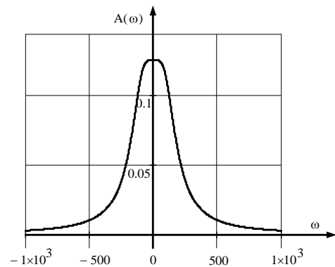
Рисунок 3– Годограф амплітудо - частотної характеристики
