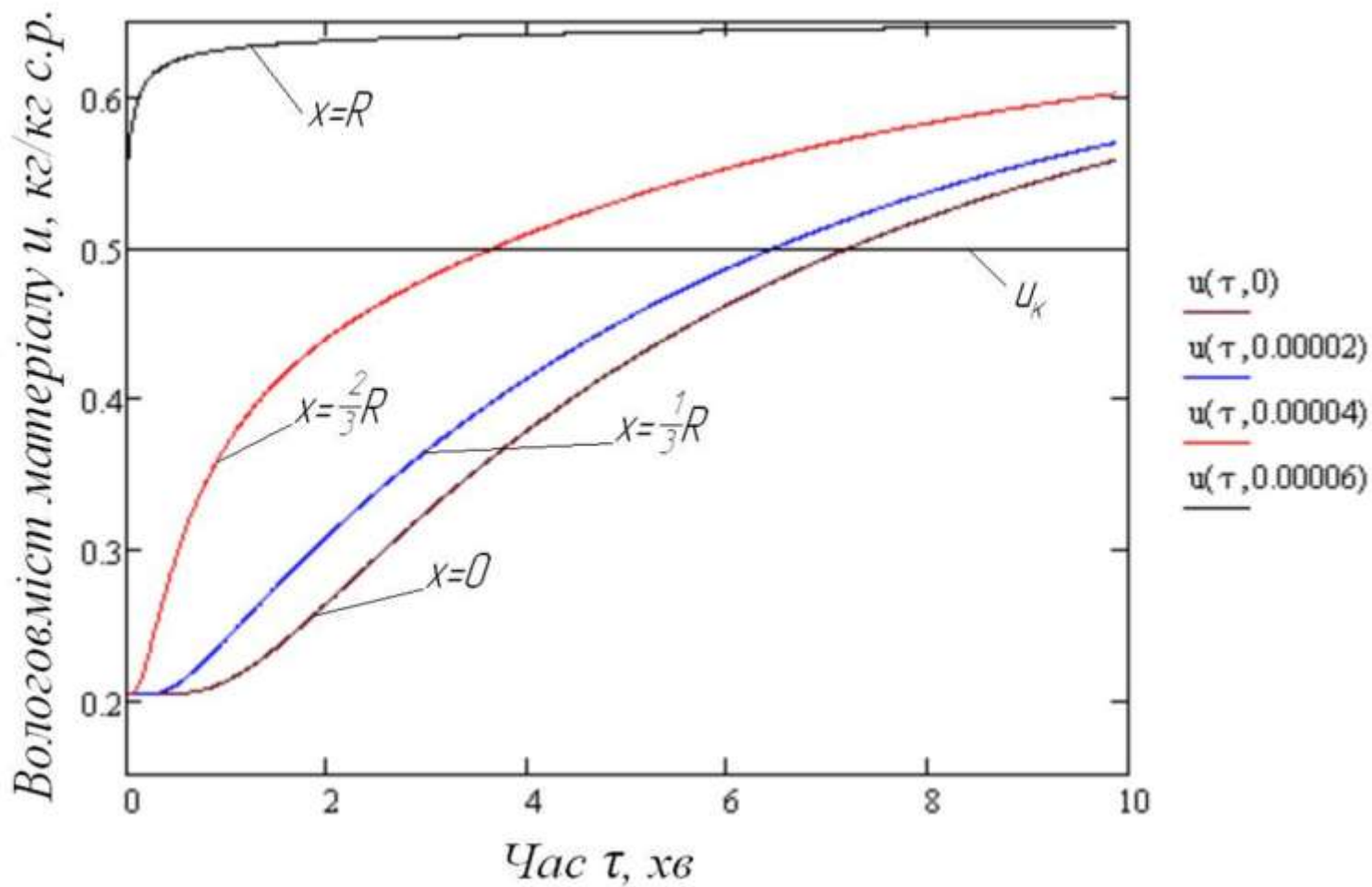
Криві зволоження листка за часом ( \tau ) і координатою ( x ) (товщиною листка)
