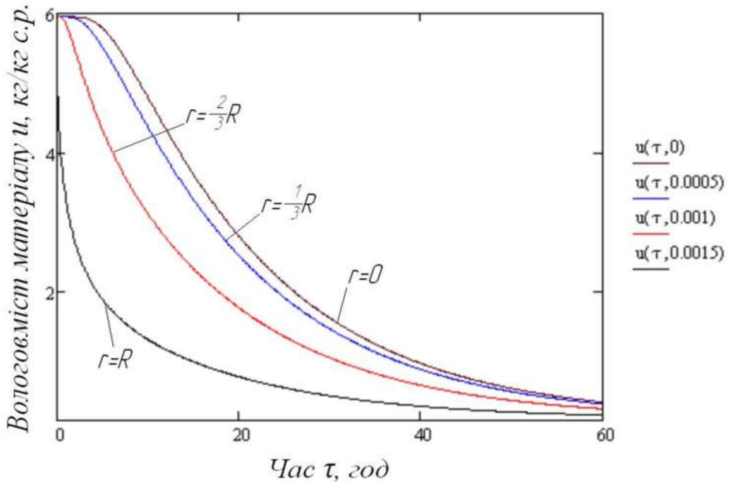
Криві сушіння листа люцерни за часом ( \tau ) і координатою ( r ) (радіусом стебла)
