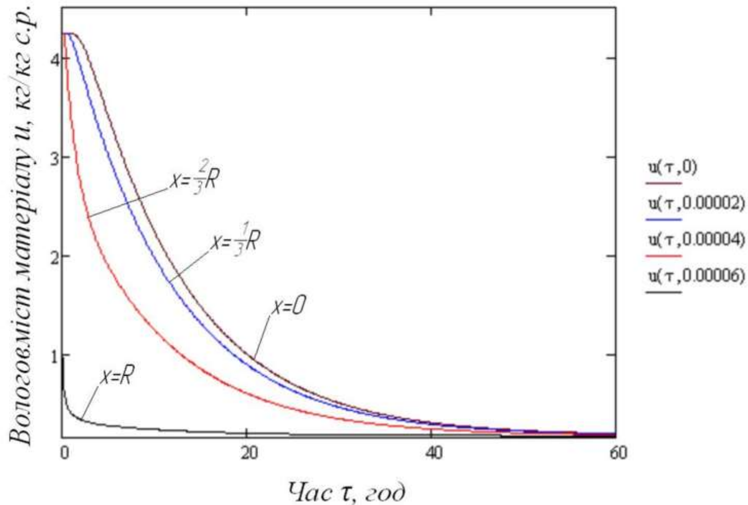
Криві сушіння листа люцерни за часом ( \tau ) і координатою ( x ) (товщиною листка)
