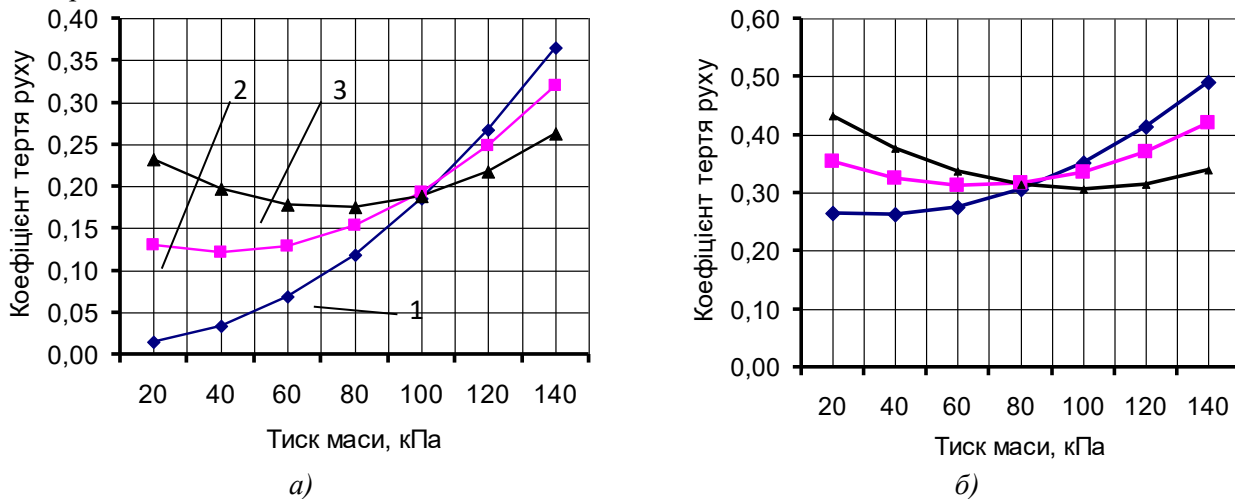
Рис. 3. Графік залежності коефіцієнта тертя руху від тиску маси для вологості люцерни 20 % (а) і 48 % (б) при швидкості обертання ножа: 1 – V = 1,0 м/с; 2 – V = 2,0 м/с; 3 – V = 3,0 м/с
