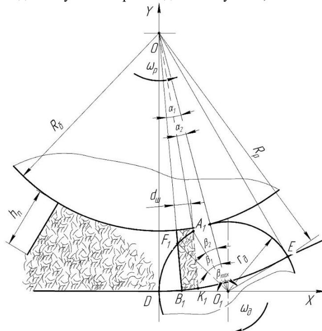
Рис. 2. Схема до визначення площі контакту трав'яної маси із поверхню дискового ножа
