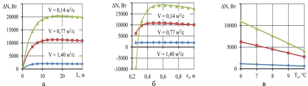
Рис. 5. Графіки залежності корисної теплової потужності тритрубного рекуператора \Delta N від його конструктивно-режимних параметрів (а - довжини зовнішнього повітропроводу; б - радіуса зовнішнього повітропроводу; в - температури навколишнього середовища)
