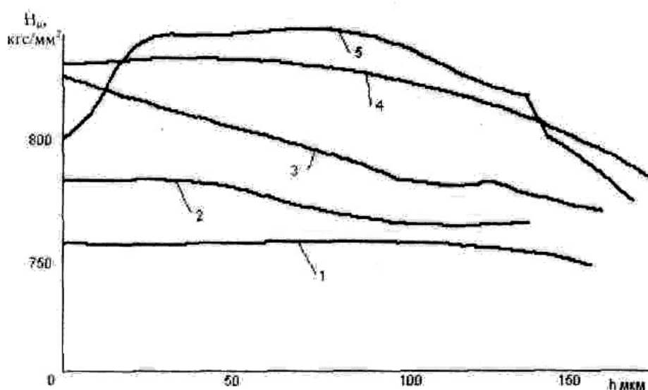
Рис.6. Изменение H_{\mu} в поверхностном слое при обработке стали 30Х3ВА при f=30 Гц: 1 – исходная; 2 – t=60 мин; 3 – t=120 мин ( A=2,5 мм); 4 – t=120 мин; 5 – t=180 мин ( A=4,5 мм)
