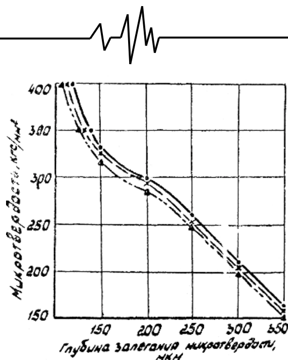
Рис. 4. Розподіл мікротвердості в поверхневому шарі сталі 45Г17Ю3 по глибині залегання [9]
