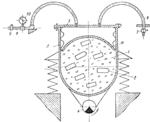
Рис. 10. Рабочий контейнер с регулируемым давлением рабочей среды:
