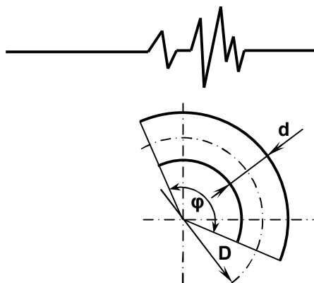
Рис. 1. Схема до визначення геометричних параметрів відводу
