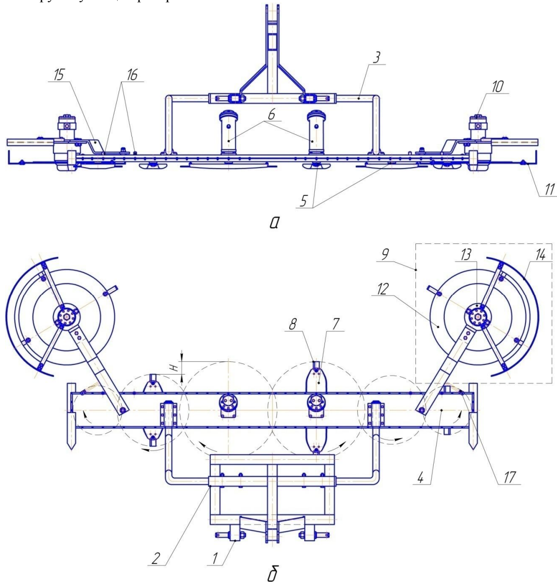
Рис. 3. Роторна косарка для мульчування пристовбурних смуг дерев в інтенсивних садах: а – вигляд з боку; б – вигляд зверху
